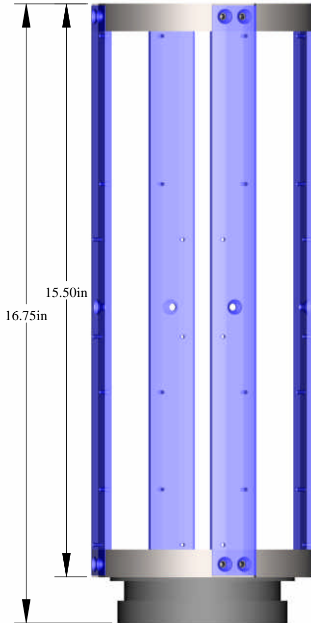
Booster Fin Frame
